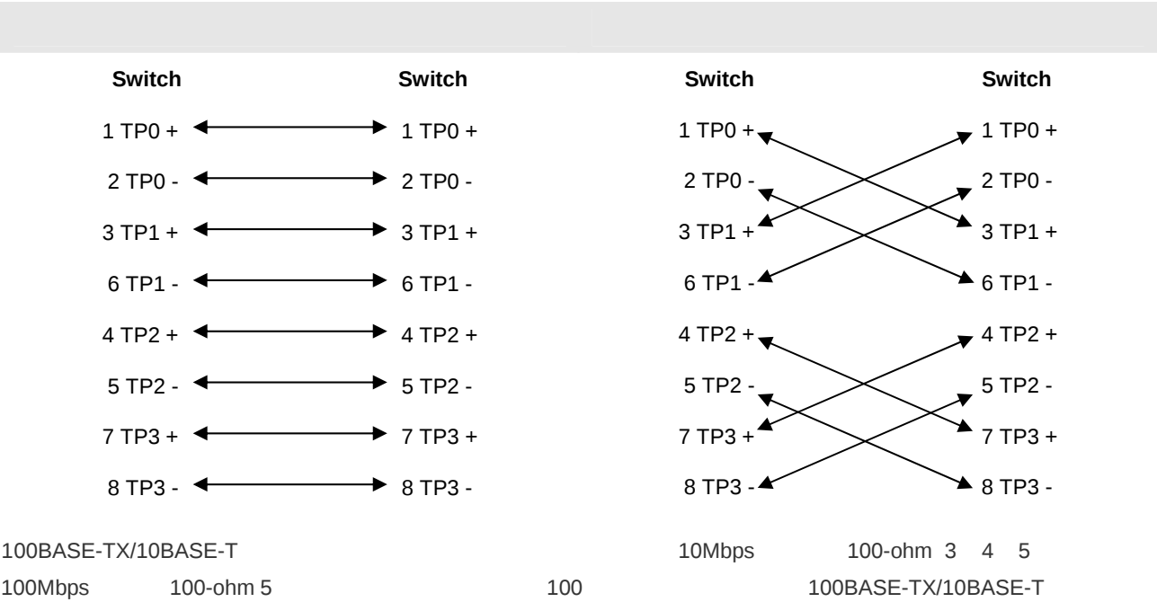
A-1 1000BASE-T
